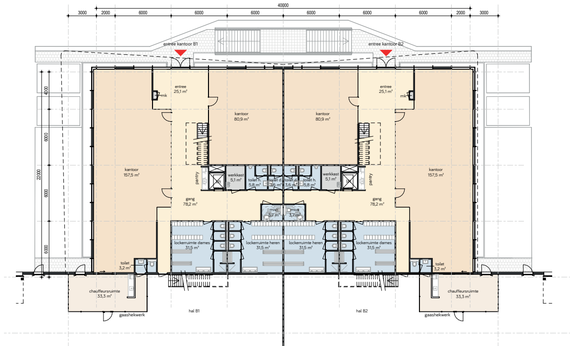
PLATTEGRONDEN KANTOOR
